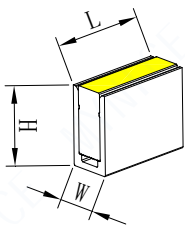
Clips & Alum. Carrier:L30*W6*H11.6 mm
